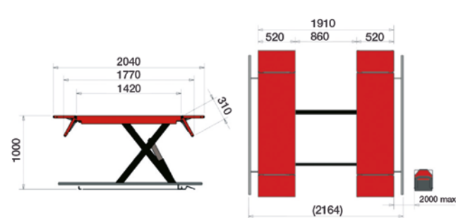
TITAN XC 1320 B
